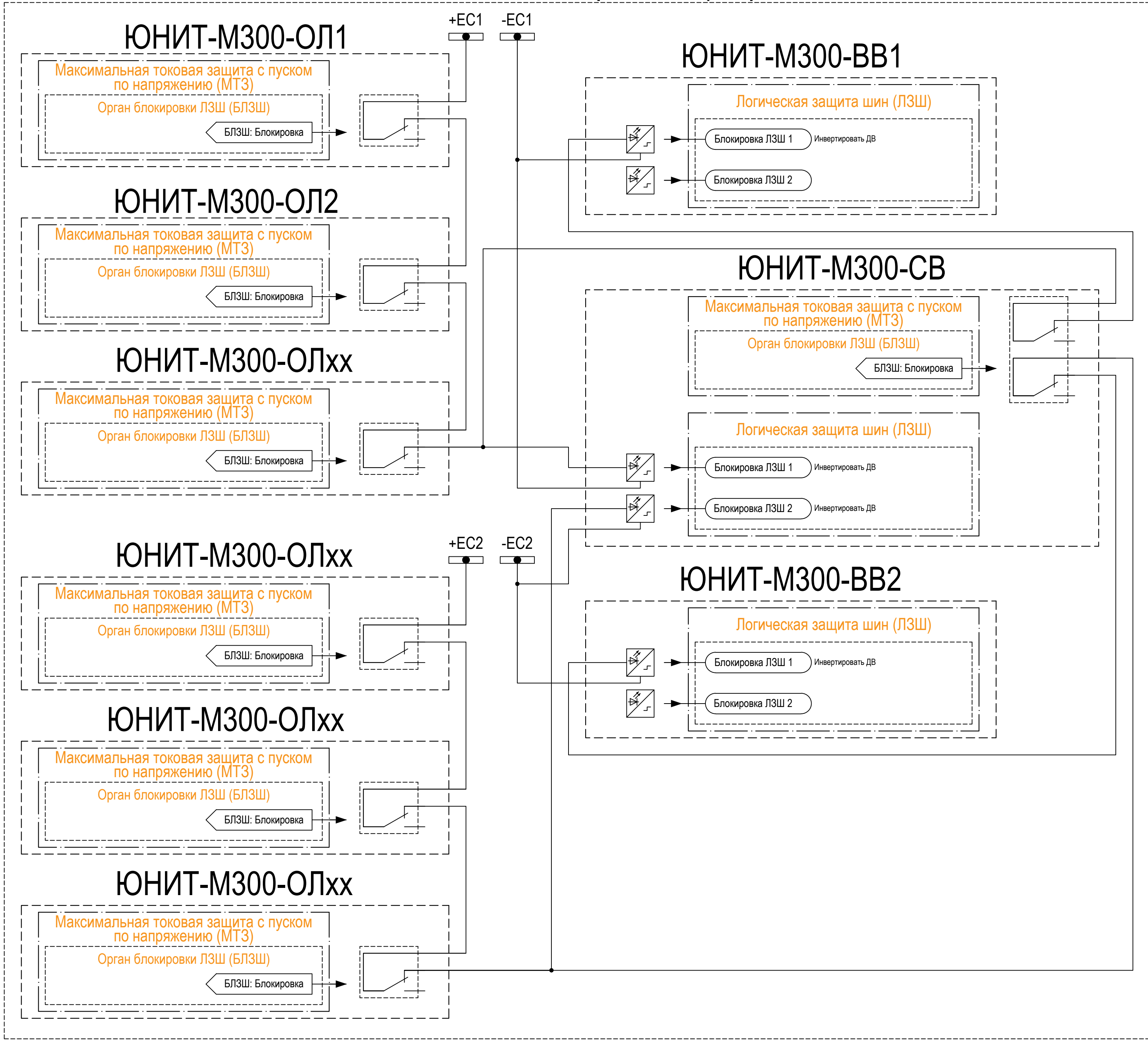
Последовательная схема организации работы ЛЗШ
