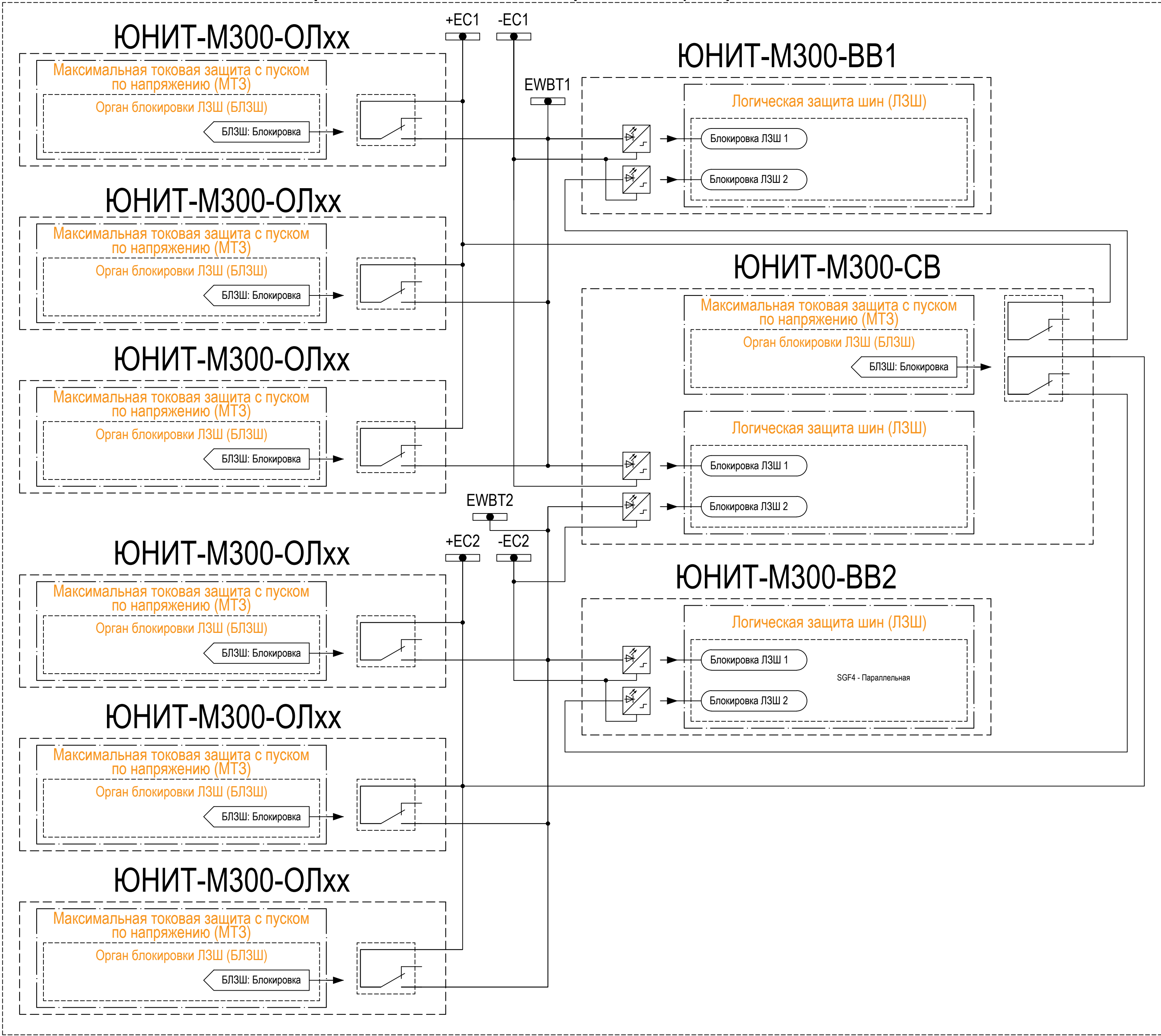
Параллельная схема организации работы ЛЗШ
